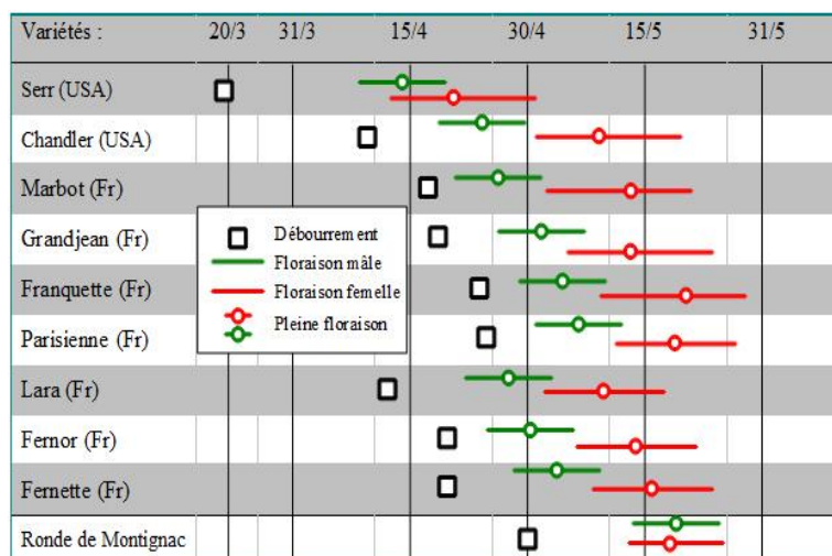
Figure 8: Echelle de précocité de débournement et de floraison mâle et femelle de 10 variétés de noyer
