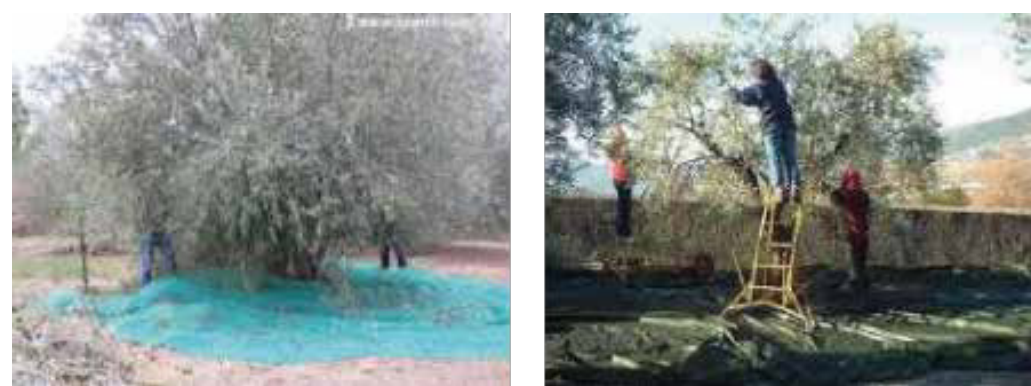
Utilisation de filets plastiques et des échelles mobiles légères dans la cueillette des olives
